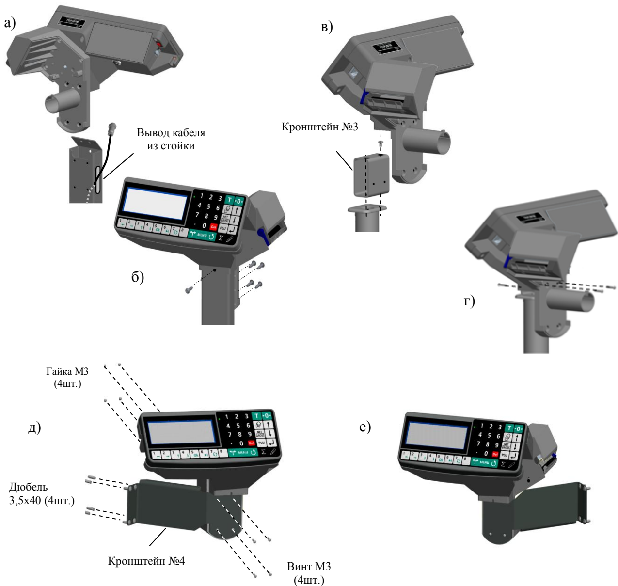
Рис. 2.2 – Варианты крепления терминалов RP и R2P: а, б – на стойке весов МК и ТВ в, г – на стойке весов 4D д, е – на стене (право- или левостороннее крепление)
